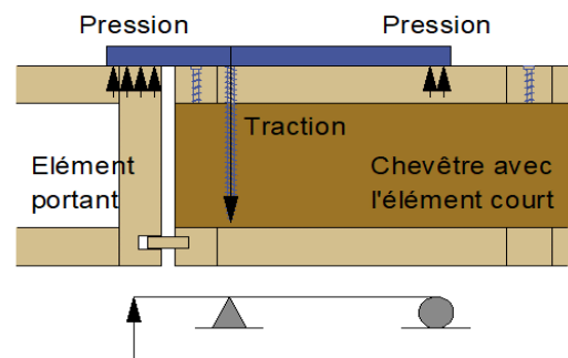
Système statique de la plaque en acier
